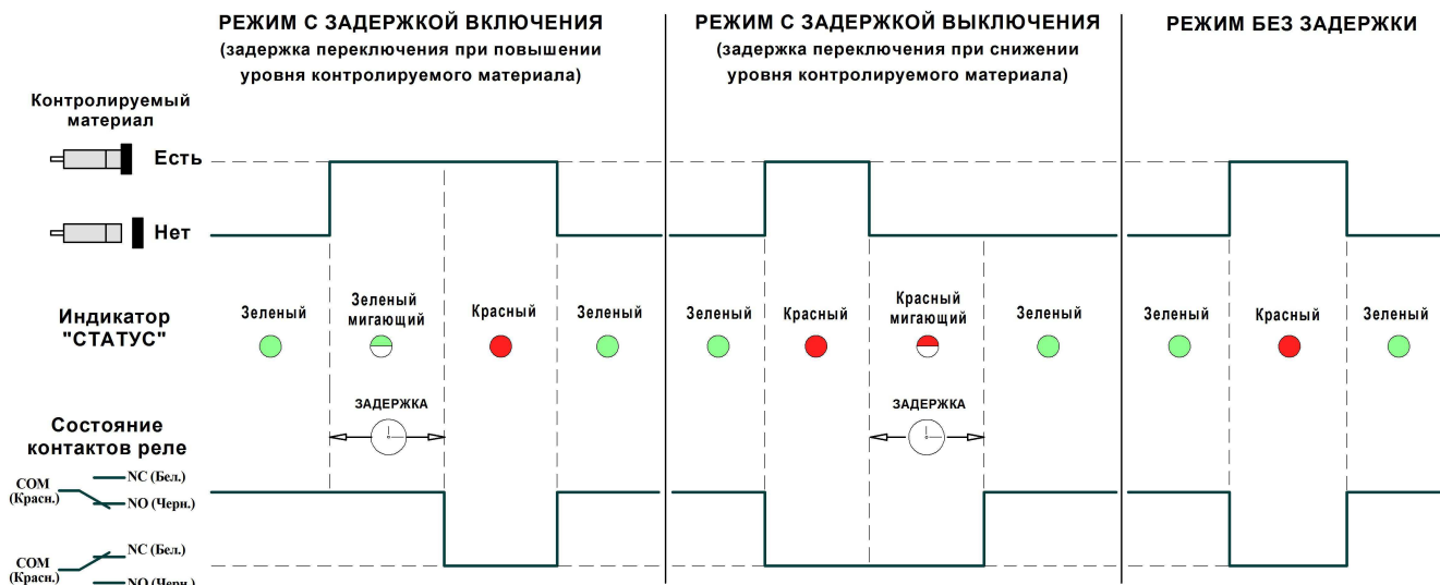
Рис.2 - Диаграммы работы датчика
